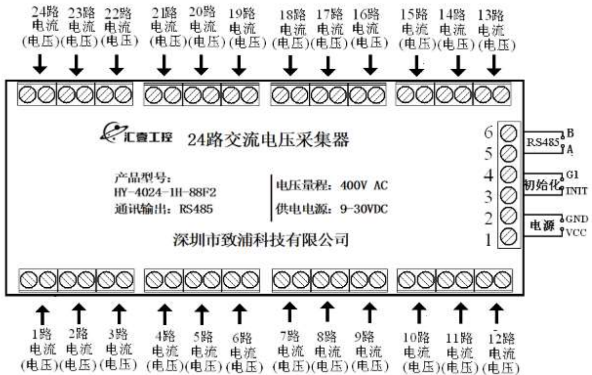
图四、产品接线参考图
