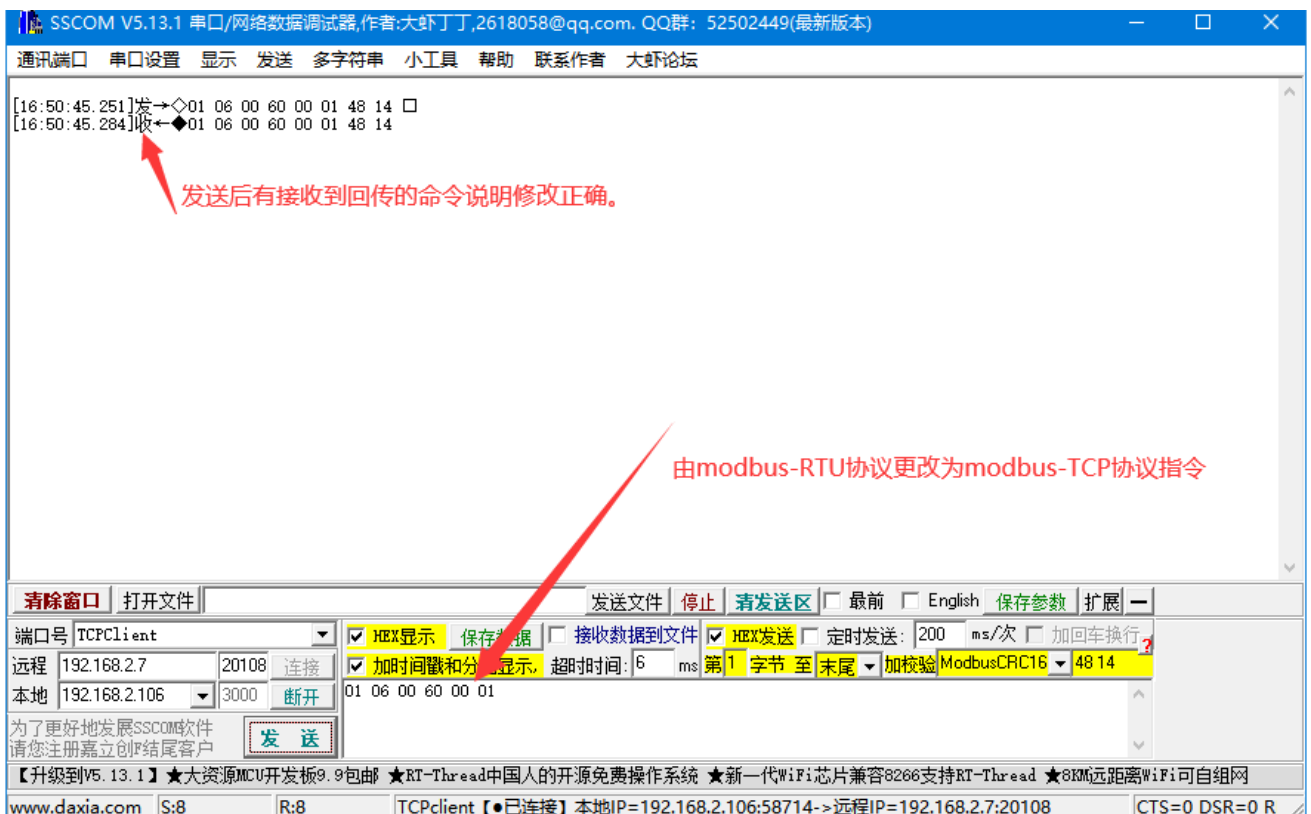
图 6、modbus-tcp 协议指令修改举例
