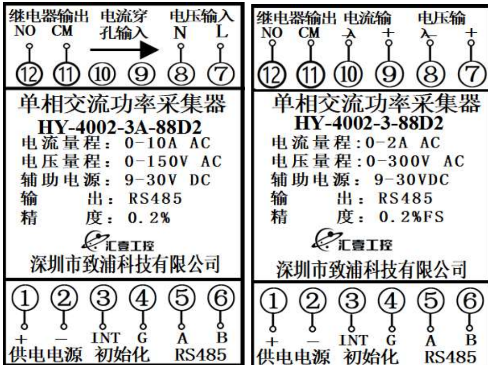
图 5.1、产品接线参考图（左图为电流穿孔输入，右图为电流 9、10 接线端子输入）
