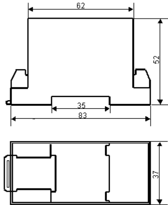
图 3.2、产品尺寸图（单位：mm）
