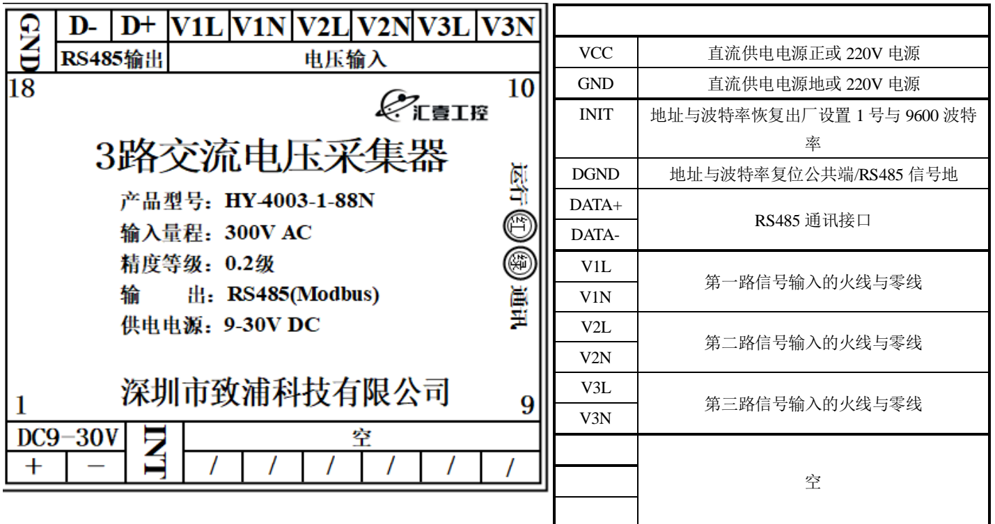
图 5.1、产品接线参考图
