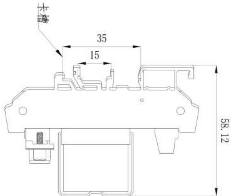
图 5.1、T0504 型正面图
