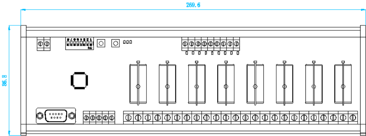
图 5.1、0808 型正面图
