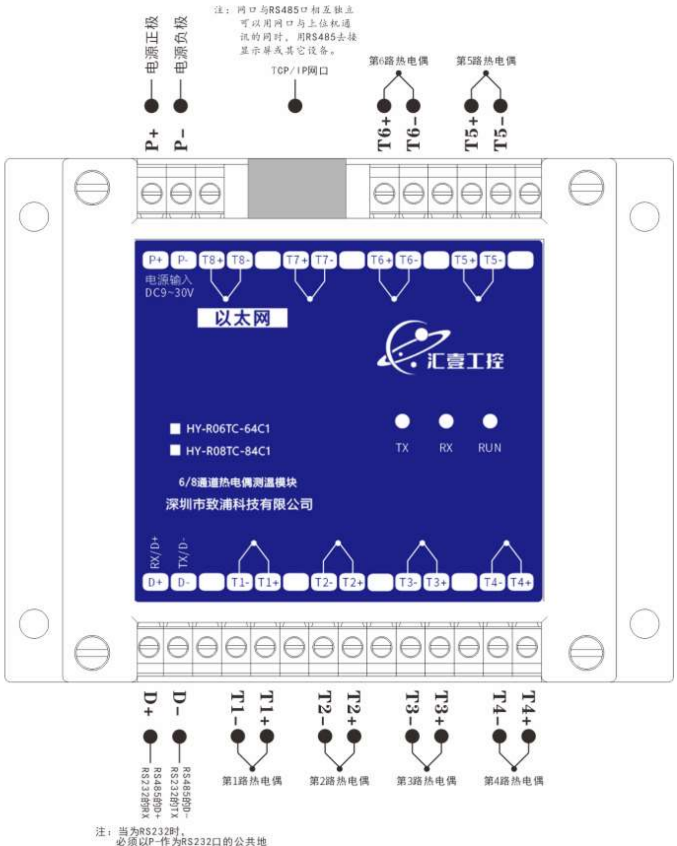
图：以太网接口版本接线图
