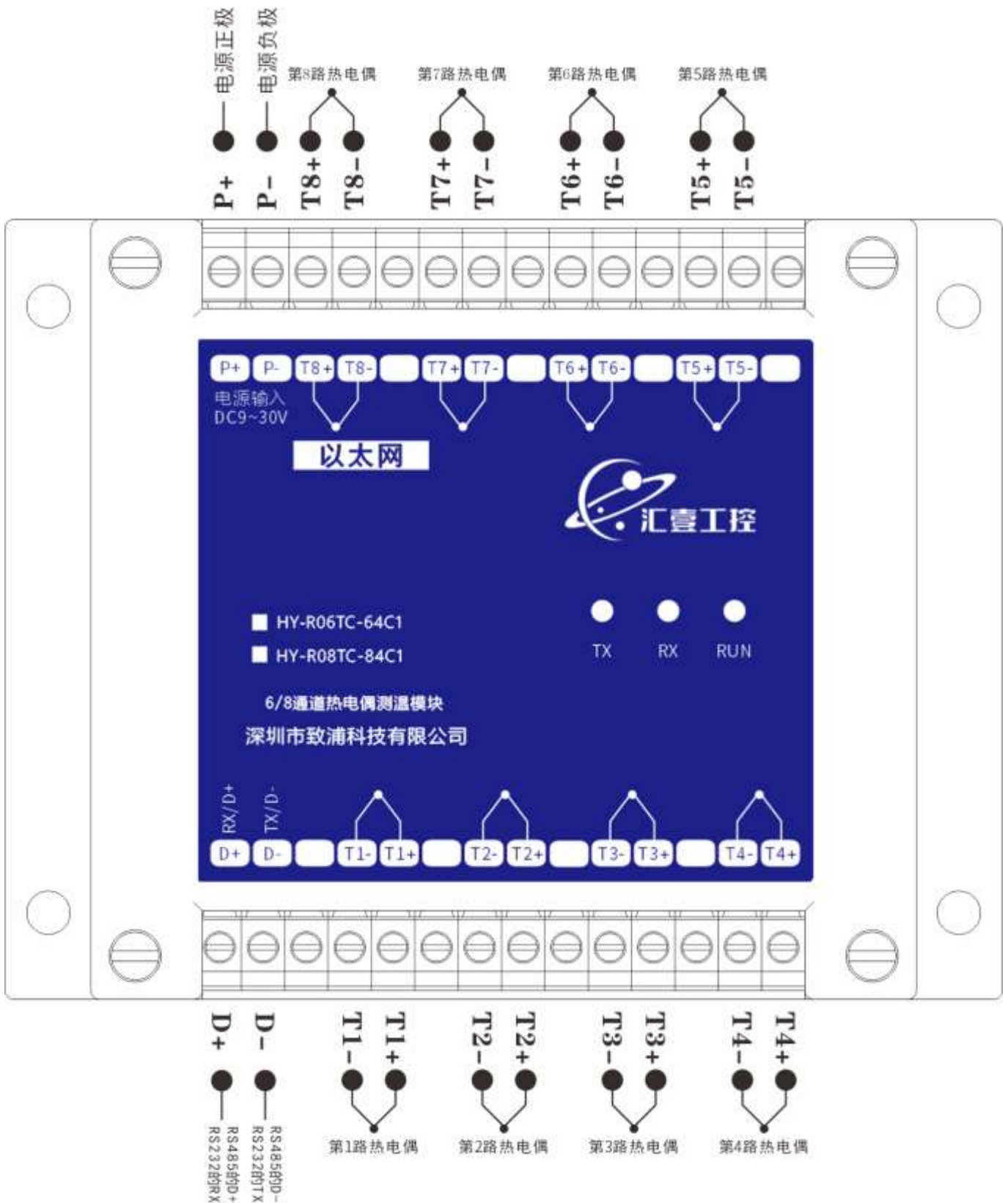
图: RS485/RS232 接口版本接线图
