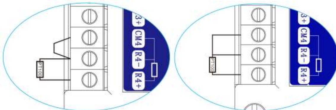
二线制接法
